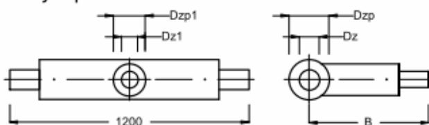
Trójnik płaski
